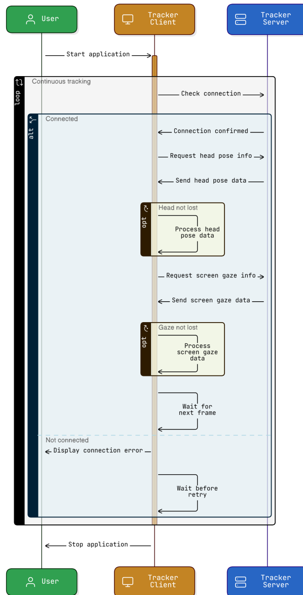
Abbildung 5: Visuelle Darstellung des Codes zur Beam SDK, Quelle: [10], [5]
