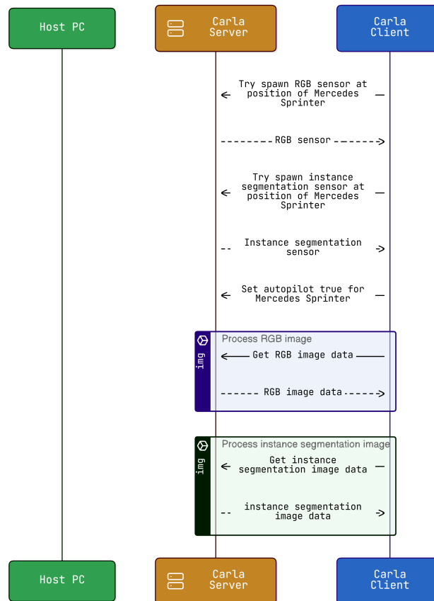
Abbildung 8: Visuelle Darstellung des Codes zur CARLA Testumgebung Teil 2/2, Quelle: [5],[13]
