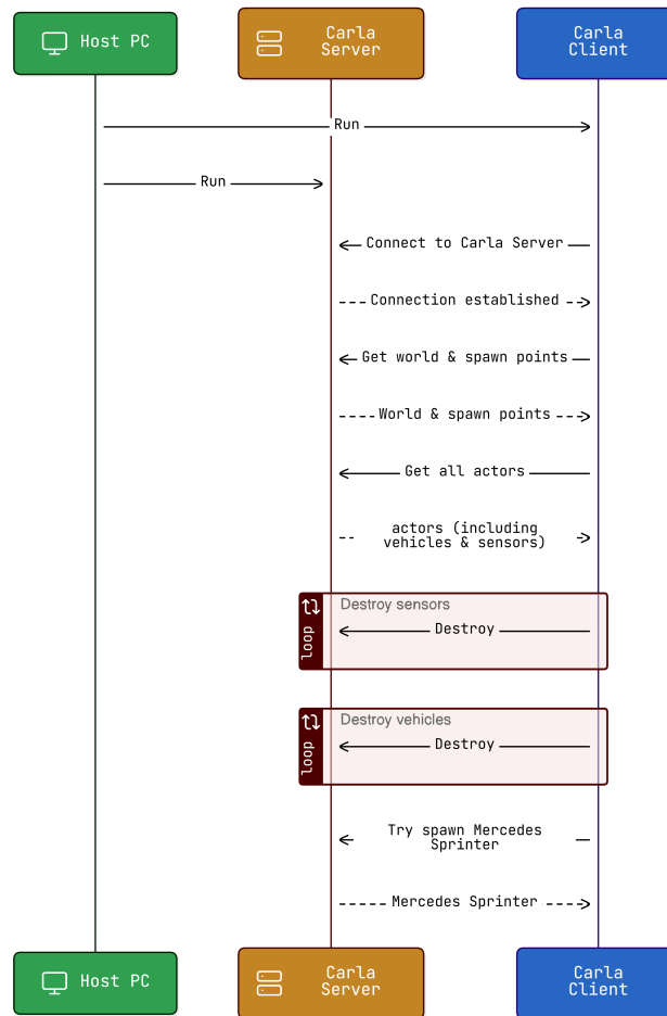
Abbildung 7: Visuelle Darstellung des Codes zur CARLA Testumgebung Teil 1/2, Quelle: [5],[13]
