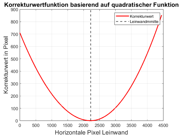
Abbildung 18: Visualisierung quadratische Korrekturfunktion, Quelle: [7]
