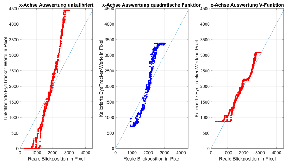
Abbildung 22: Gegenüberstellung reale Blickposition und Eye Tracker-Werte: unkalibriert (links), kalibriert quadratische Funktion (mitte), kalibriert V-Funktion (rechts), Quelle: [7]
