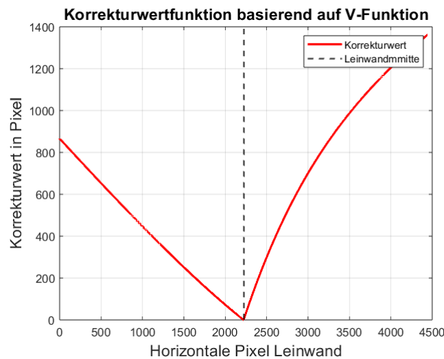
Abbildung 21: Visualisierung V-Korrekturfunktion, Quelle: [7]
